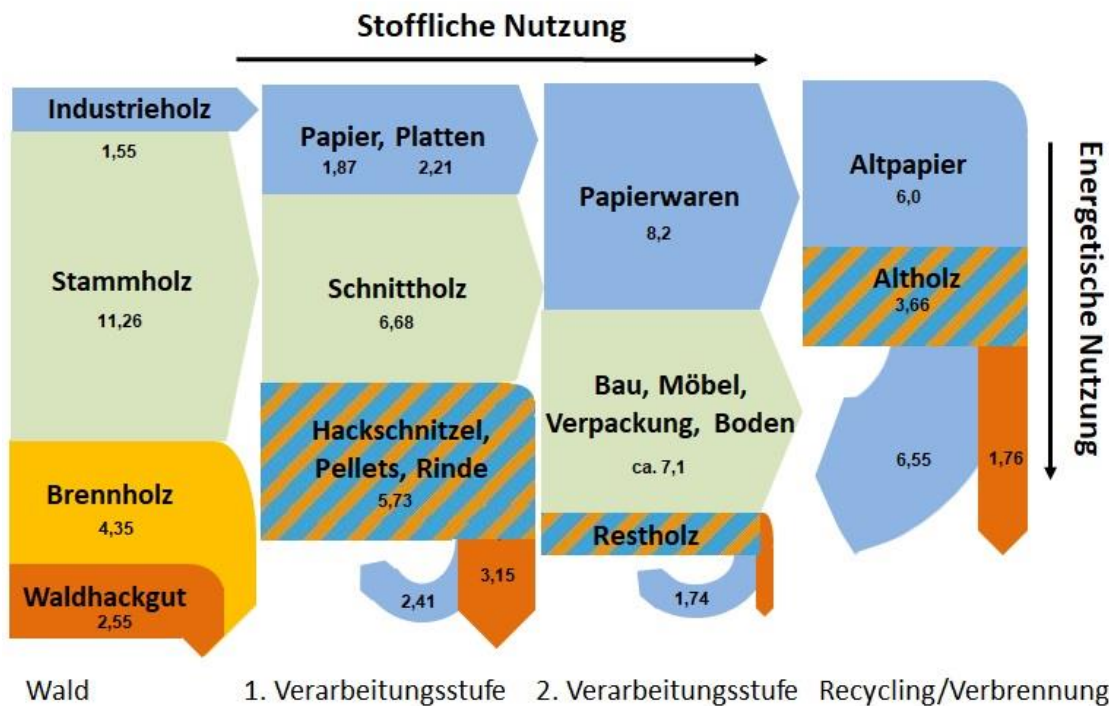
Abbildung 45: Die Stoffströme der stofflichen und energetischen Holzverwendung in Bayern 2018 in Mio. Fm m. R. bzw. m³ in einer vereinfachten Darstellung.
