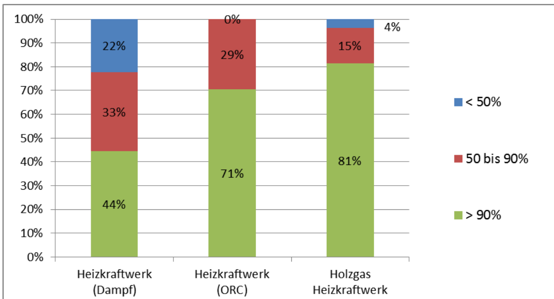
Abbildung 37: Verteilung des Wärmenutzungsgrades bei Biomasse(heiz)kraftwerken, ungewichtet (C.A.R.M.E.N.-Umfrage 2019, Heizkraftwerke (Dampf) n=18, Heizkraftwerke (ORC) n=17, Holzgas Heizkraftwerk n=27)
