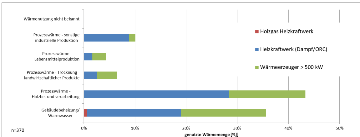
Abbildung 33: Art der Wärmenutzung und deren Anteil an der genutzten Wärmemenge (C.A.R.M.E.N.-Umfrage 2019/2016, Wärmeerzeuger > 500 kW n=286, Heizkraftwerke (Dampf/ORC) n=57, Holzgas Heizkraftwerk n=27)
