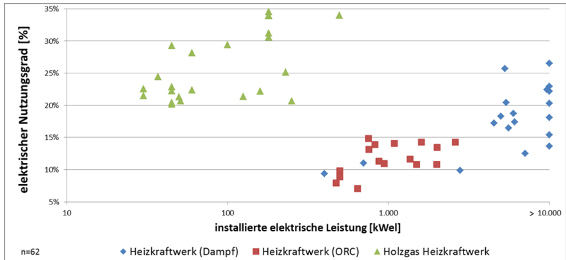
Abbildung 36: Verteilung der elektrischen Nutzungsgrade in Abhängigkeit der installierten Leistung und Verstromungstechnologie (C.A.R.M.E.N.-Umfrage 2019, n=62)
